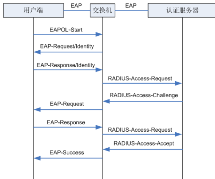
图 13-21 EAP-MD5 认证过程
