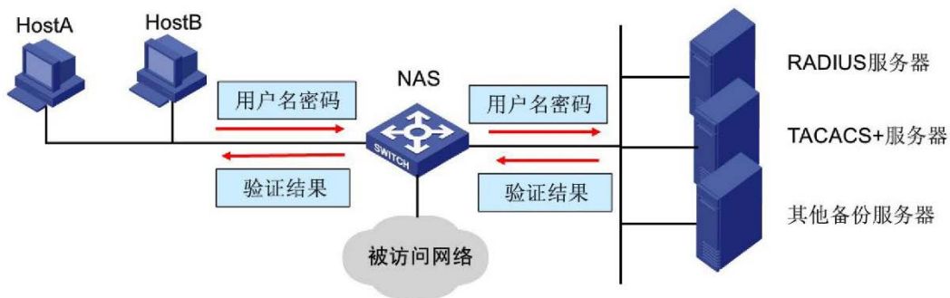
图 13-25 AAA 架构
