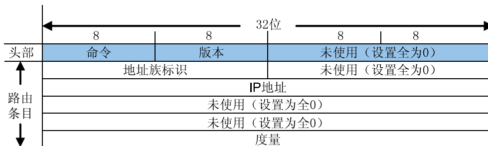
图 10-31 RIPv1 的报文格式
