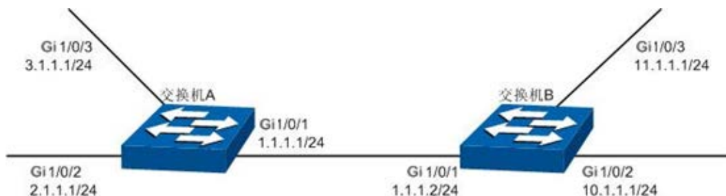
图 10-37 组网图
