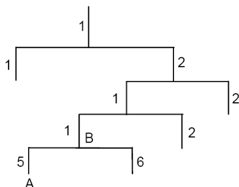
图 14-2 MIB 树结构
